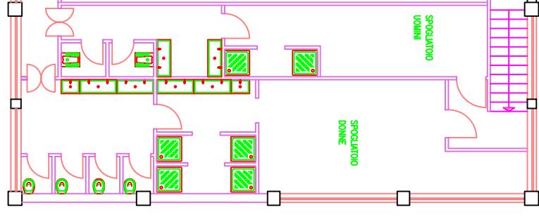
PROGETTO PIANTA PIANO SOPPALCO
